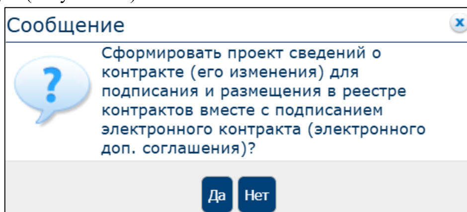
Рисунок 135. Информационное сообщение
