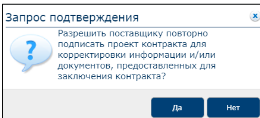
Рисунок 132. Запрос подтверждения
